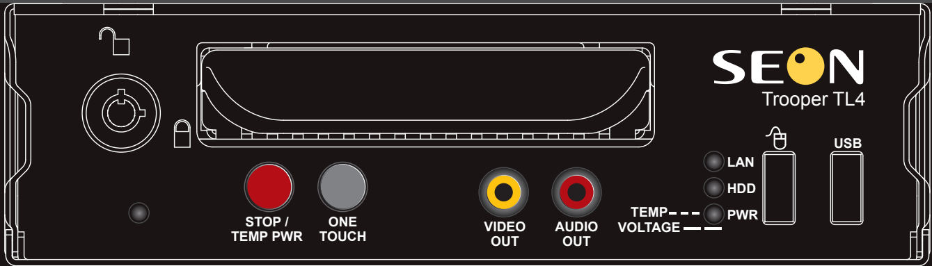
Trooper® TL4 front panel – actual size
